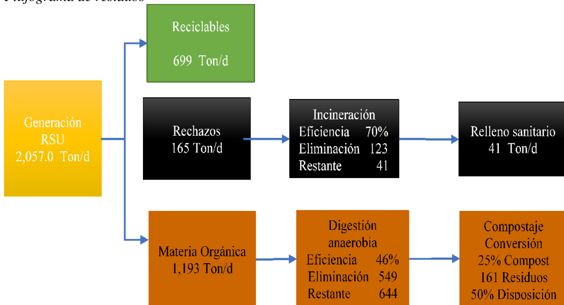
Figura 3 Flujograma de residuos
